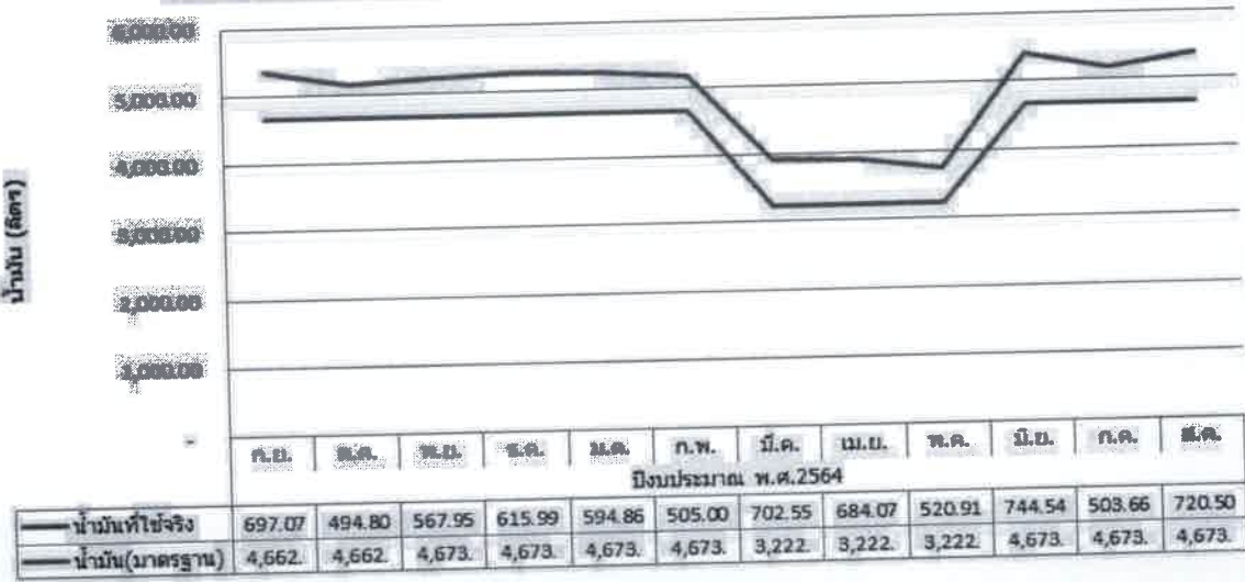
กราฟแสดงการใช้พลังงานเชื้อเพลิง ปีงบประมาณ พ.ศ.๒๕๖๔
